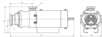
Mått HYGHSPIN Extended fri axial (mm)
